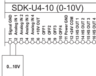
Ansteuerung mit externer Spannungsquelle
