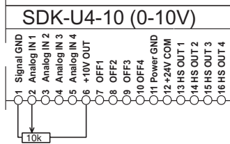
Ansteuerung mit Standardpoti
