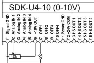
Ausschalten mit Arbeitskontakt Ein = Arbeitskontakt offen
