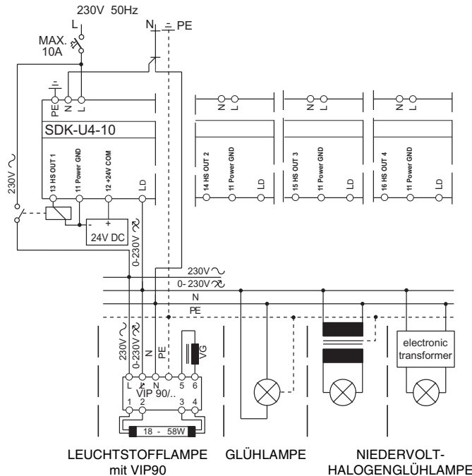
Ausschalten mit Arbeitskontakt Ein = Arbeitskontakt offen
