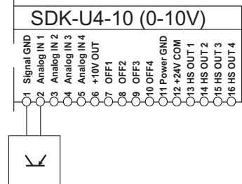
Ansteuerung mit Sinkstromquelle (z.B. EIB)
