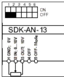
Ansteuerung mit Standardpoti
