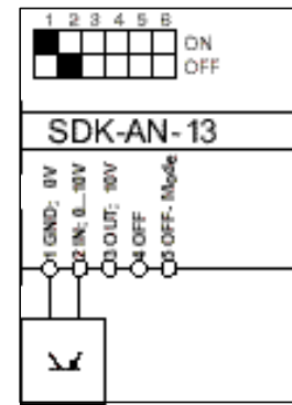
Ansteuerung mit Sinkstromquelle (z.B. EIB)
