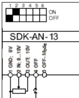
Kontakt offen = Ein Kontakt geschlossen = Aus
