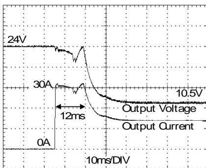
Bild 23-3 30A Spitzenlast, typ.
