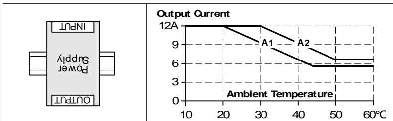
Bild 23-6 Einbaulage B (Auf dem Kopf stehend)
