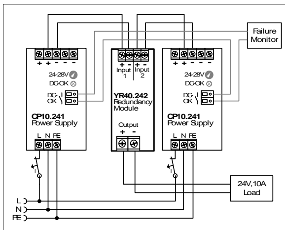
Bild 22-1 Typische 1+1 redundante Verschaltung für 10A mit dem Redundanzmodul YR40.242 MOSFET
