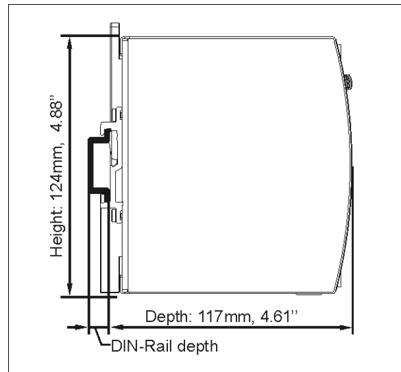
Bild 21-3 Seitenansicht
