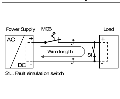
Bild 23-4 Prüfschaltung
