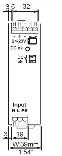
Bild 21-2 Frontansicht CP10.241-S1
