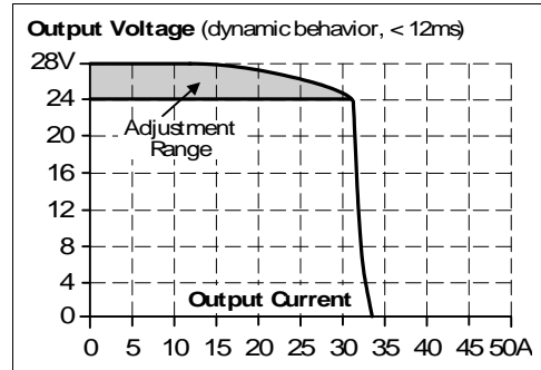
Bild 6-2 Dynamische Ausgangsstromfähigkeit, typ.
