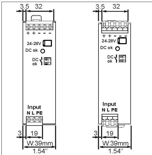
Bild 21-1 Frontansicht CP10.241, CP10.242
