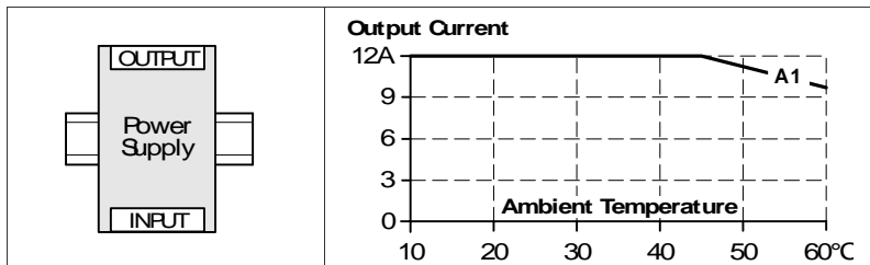
Bild 23-5 Einbaulage A (Standard- Einbaulage)
